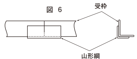
山形鋼
